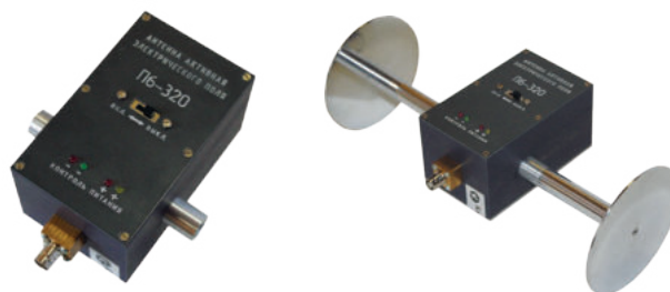
Антенна П6-320.
