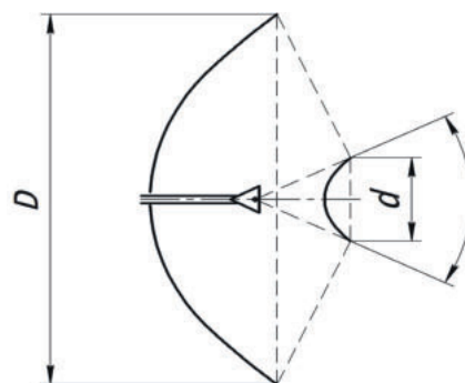
Схема зеркальной антенной системы ЗА6-1,2.
