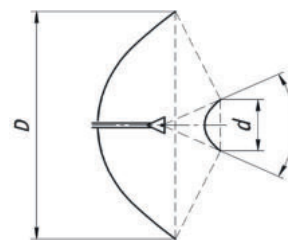
Схема зеркальной антенной системы РЗА4-0,9.
