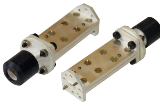
Модель облучающей системы для различных участков диапазона.
