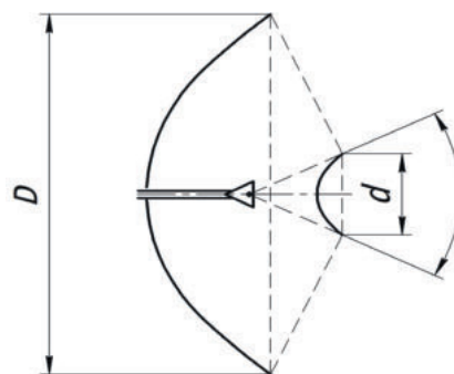
Схема зеркальной антенной системы ЗА5-0,4.
