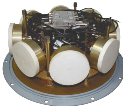
Антенная система АСКМ 1/8-0,9/18 на шасси.
