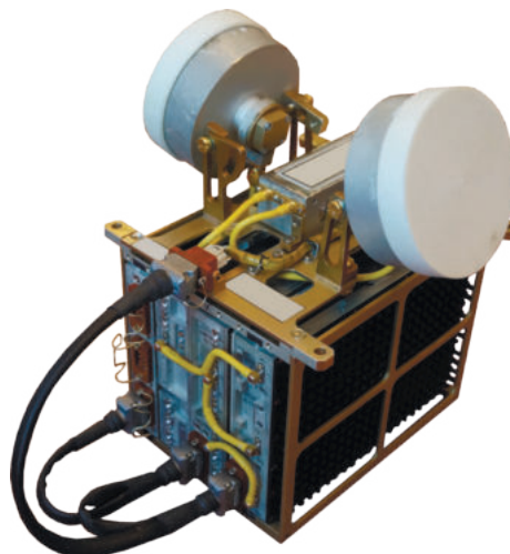
2-канальный преобразователь частоты диапазона 0,9 - 18 ГГц, серии Универсал-1, комплексированный с антенной системой.
